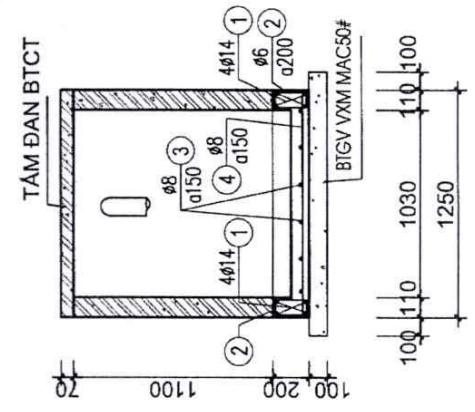
CẮT 2-2
